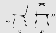
SILLA DURBAN 4514 CARCASA MADERA PATA REDONDA METÁLICA Ø 25 ROUND METAL LEGS Ø 25 PIEDS MÉTAL RONDE Ø 25
