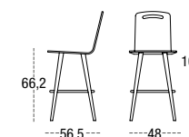
TABURETE MEDIO DURBAN 6511 CARCASA MADERA PATA MADERA CUADRADA SQUARE WOODEN LEGS PIEDS BOIS CARRE
