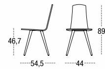
SILLA BONN 4502 CARCASA TAPIZADA PATA MADERA REDONDA ROUND WOODEN LEGS PIEDS BOIS RONDE
