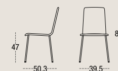
SILLA BELICE 4541 CARCASA TAPIZADA PATA CUADRADA METÁLICA SQUARE METAL LEGS PIEDS MÉTAL CARRE
