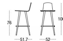
TABURETE ALTO NEUSS 7521 CARCASA MADERA PATA MADERA CUADRADA SQUARE WOODEN LEGS PIEDS BOIS CARRÉ
