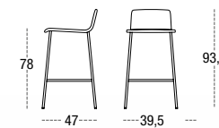
TABURETE ALTO DURERO 7551 CARCASA TAPIZADA PATA CUADRADA METÁLICA SQUARE METAL LEGS PIEDS MÉTAL CARRE
