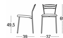
TABURETE BAJO YOLANDA 45 PATA METÁLICA CUADRADA SQUARE METAL LEGS PIEDS MÉTAL CARRE
