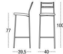
TABURETE ALTO ALOHA 75 ASIENTO 33 cm PATA CUADRADA METÁLICA SQUARE METAL LEGS PIEDS MÉTAL CARRÉ
