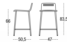
TABURETE MEDIO DURERO 6552 CARCASA MADERA PATA CUADRADA MADERA SQUARE WOODEN LEGS PIEDS BOIS CARRE
