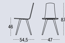
SILLA BONN 4501 CARCASA TAPIZADA PATA MADERA CUADRADA SQUARE WOODEN LEGS PIEDS BOIS CARRE
