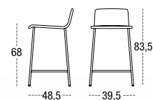
TABURETE MEDIO DURERO 6551 CARCASA TAPIZADA PATA CUADRADA METÁLICA SQUARE METAL LEGS PIEDS MÉTAL CARRE
