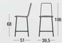
TABURETE MEDIO BELICE 6541 CARCASA TAPIZADA PATA CUADRADA METÁLICA SQUARE METAL LEGS PIEDS MÉTAL CARRÉ
