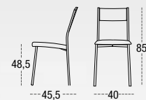
SILLA LUBA PATA CUADRADA METÁLICA SQUARE METAL LEGS PIEDS MÉTAL CARRÉ
