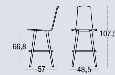
TABURETE MEDIO BONN 6501 CARCASA TAPIZADA PATA MADERA CUADRADA SQUARE WOODEN LEGS PIEDS BOIS CARRE
