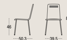
SILLA BELICE 4541 CARCASA MADERA PATA CUADRADA METÁLICA SQUARE METAL LEGS PIEDS MÉTAL CARRE
