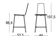
TABURETE MEDIO BONN 6503 CARCASA TAPIZADA PATA REDONDA METÁLICA Ø 18 ROUND METAL LEGS Ø 18 PIEDS MÉTAL RONDE Ø 18
