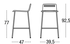
TABURETE ALTO DURERO 7551 CARCASA MADERA PATA CUADRADA METÁLICA SQUARE METAL LEGS PIEDS MÉTAL CARRE
