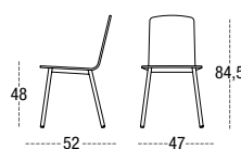
SILLA DURBAN 4514 CARCASA TAPIZADA PATA REDONDA METÁLICA Ø 25 ROUND METAL LEGS Ø 25 PIEDS MÉTAL RONDE Ø 25
