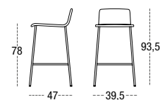
TABURETE ALTO DURERO 7551 CARCASA TAPIZADA PATA CUADRADA METÁLICA SQUARE METAL LEGS PIEDS MÉTAL CARRE
