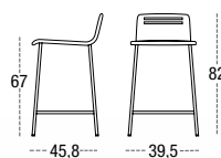
TABURETE MEDIO DURERO 6551 CARCASA MADERA PATA CUADRADA METÁLICA SQUARE METAL LEGS PIEDS MÉTAL CARRE
