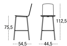
TABURETE ALTO DURBAN 7513 CARCASA TAPIZADA PATA REDONDA METÁLICA Ø 18 ROUND METAL LEGS Ø 18 PIEDS MÉTAL RONDE Ø 18
