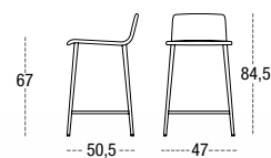
TABURETE MEDIO DURERO 6552 CARCASA TAPIZADA PATA CUADRADA MADERA SQUARE WOODEN LEGS PIEDS BOIS CARRE
