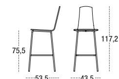
TABURETE ALTO BONN 7503 CARCASA MADERA PATA REDONDA METÁLICA Ø 18 ROUND METAL LEGS Ø 18 PIEDS MÉTAL RONDE Ø 18
