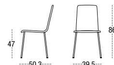
SILLA BELICE 4541 CARCASA TAPIZADA PATA CUADRADA METÁLICA SQUARE METAL LEGS PIEDS MÉTAL CARRE
